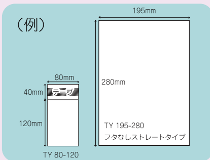
NO.40 タイプ① 規格表 (一般テープ)
